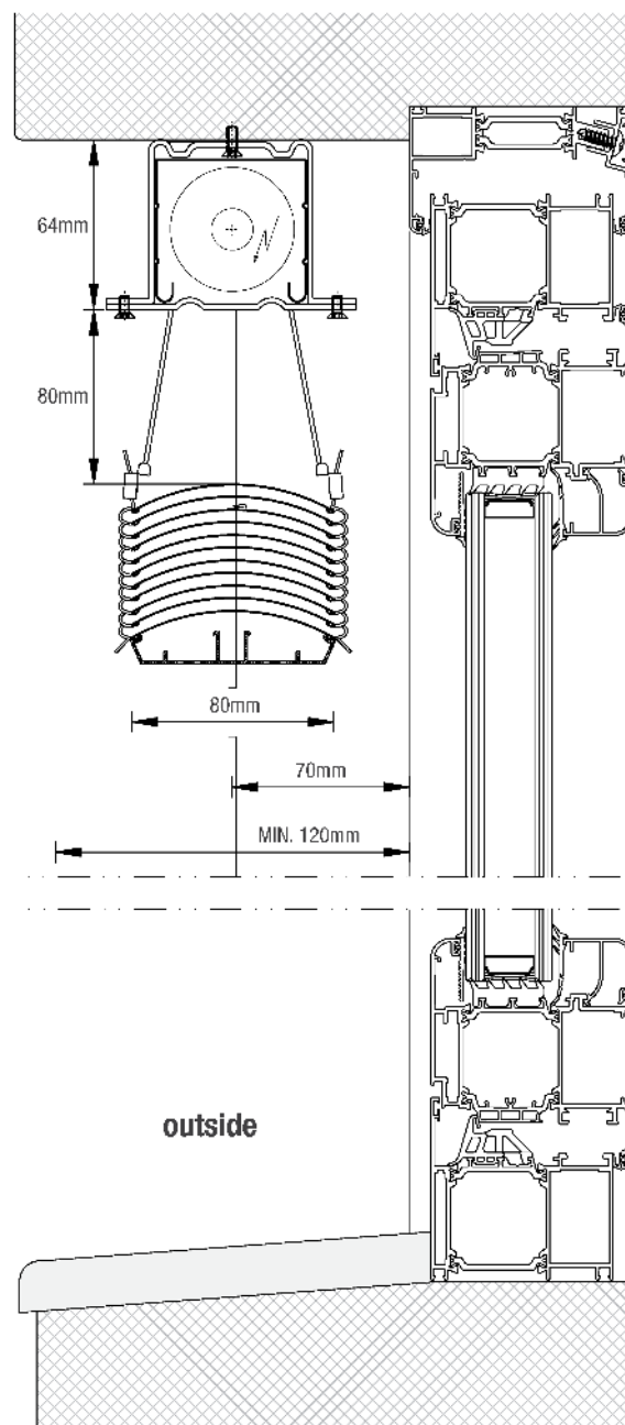
Sezione vano finestra con tenda esterna a lamelle della linea OVERSUN
