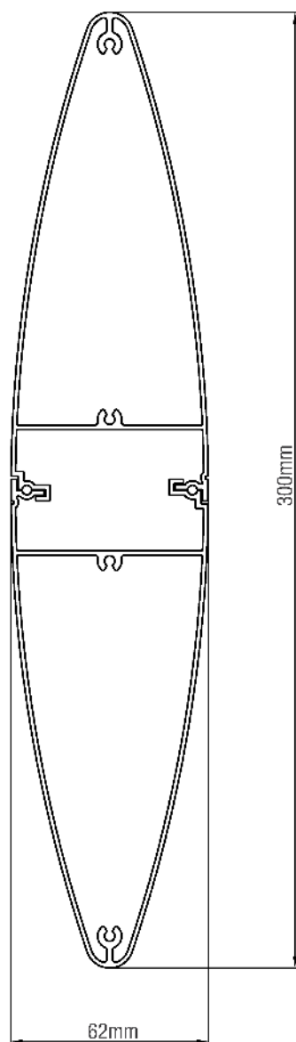
Sezione Frangisole OVERSUN modello F1 300mm
